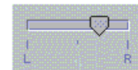
JSlider
