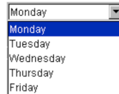
JComboBox
