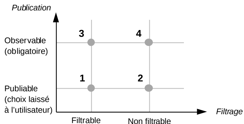
Figure 12 Quatre niveaux d'observabilité [Laurillau 1999a]
